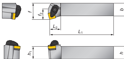
Увеличенный вид державки типа 2020
